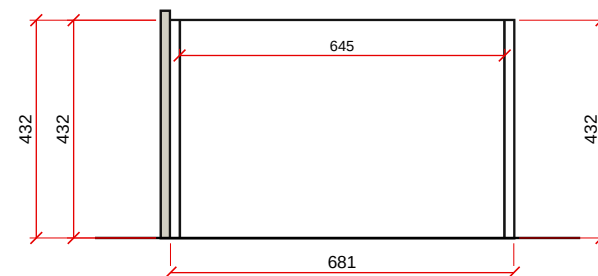
VISTA F - ESC. 1:15
