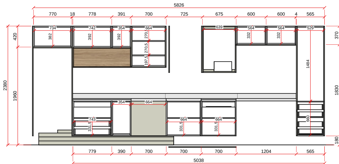
VISTA A - ESC. 1:40
