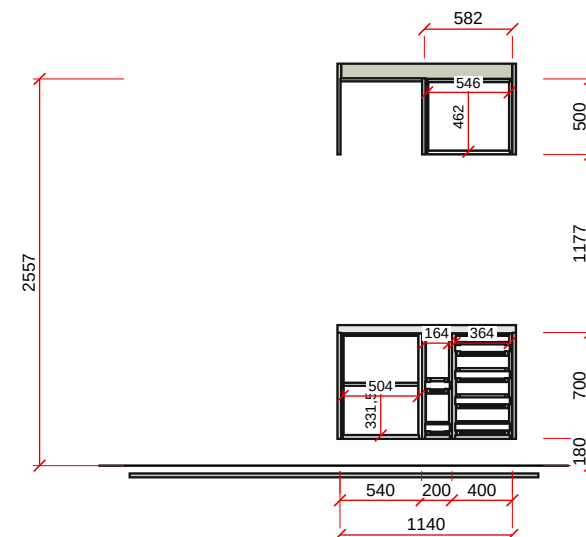
VISTA B - ESC. 1:50
