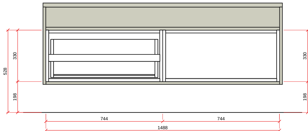
VISTA E - ESC. 1:12.5
