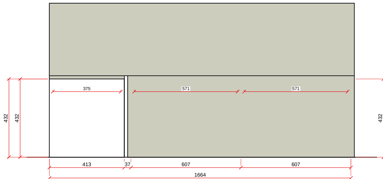
VISTA C - ESC. 1:12.5
